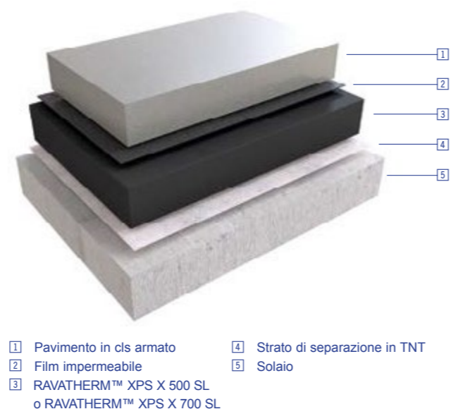
Fig. 03 Pavimenti industriali isolati con RAVATHERM™ XPS X 500/700 SL
