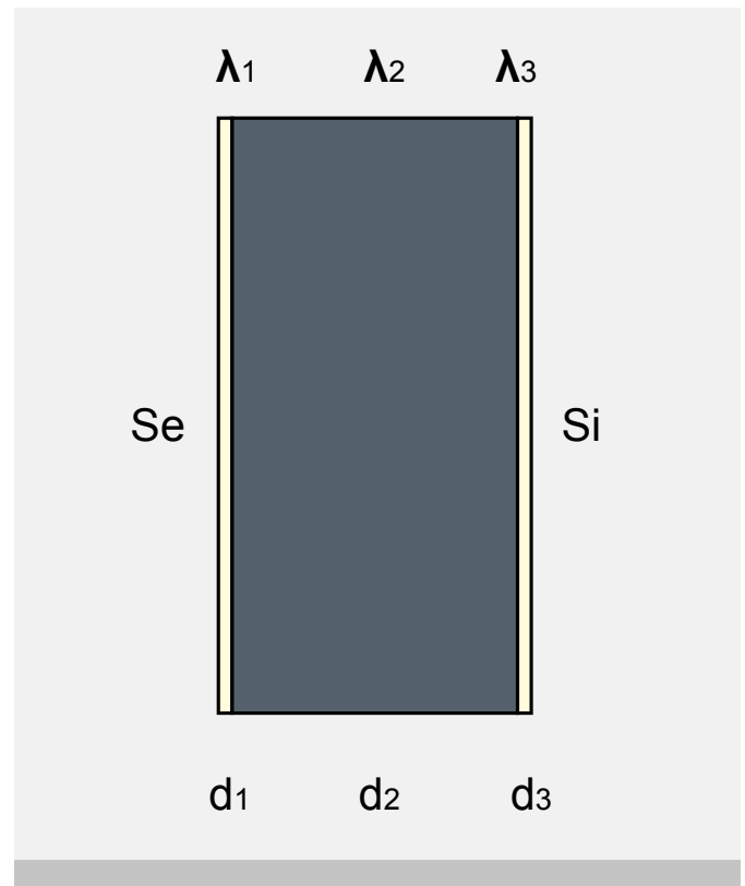
Abb. 07: Querschnitt eines 3-lagigen Sandwich-Panels
