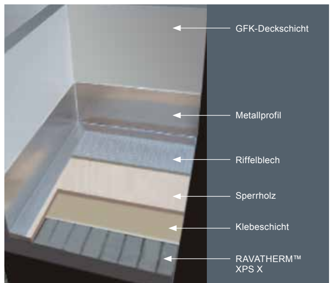
Abb. 02: Querschnitt eines Wand-/Bodenelements
